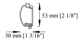
Hembar
