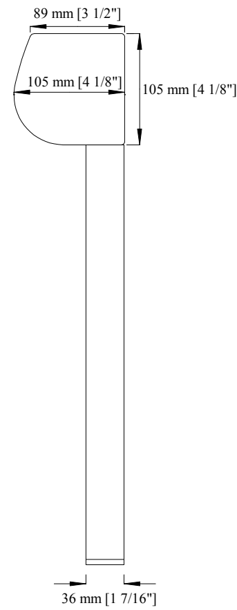
End Cap
