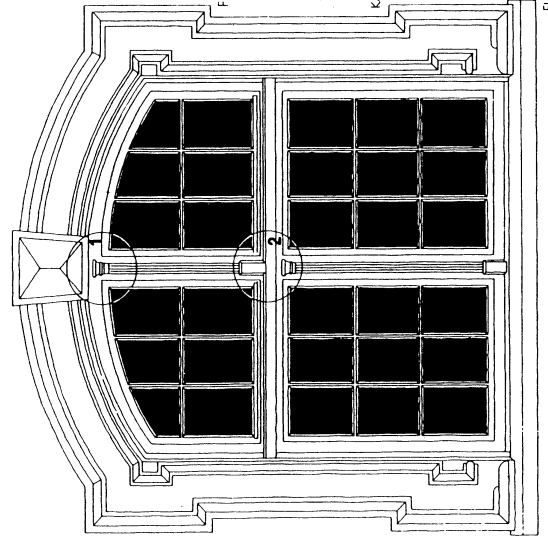
UNTERE FENSTERREIHE DES RATHAUSES IN PAPENBURG M 1 20
