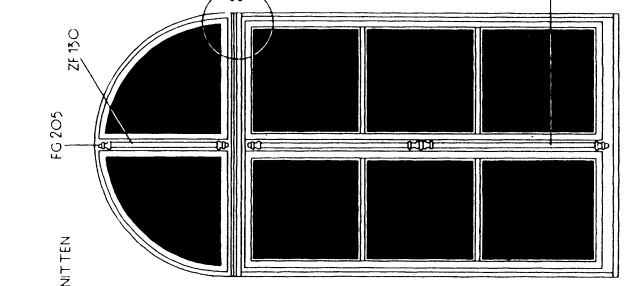
RUNDBOGENFENSTER M 1 20
